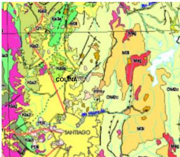
Imagen N°6: Formaciones geológicas comuna de Colina
