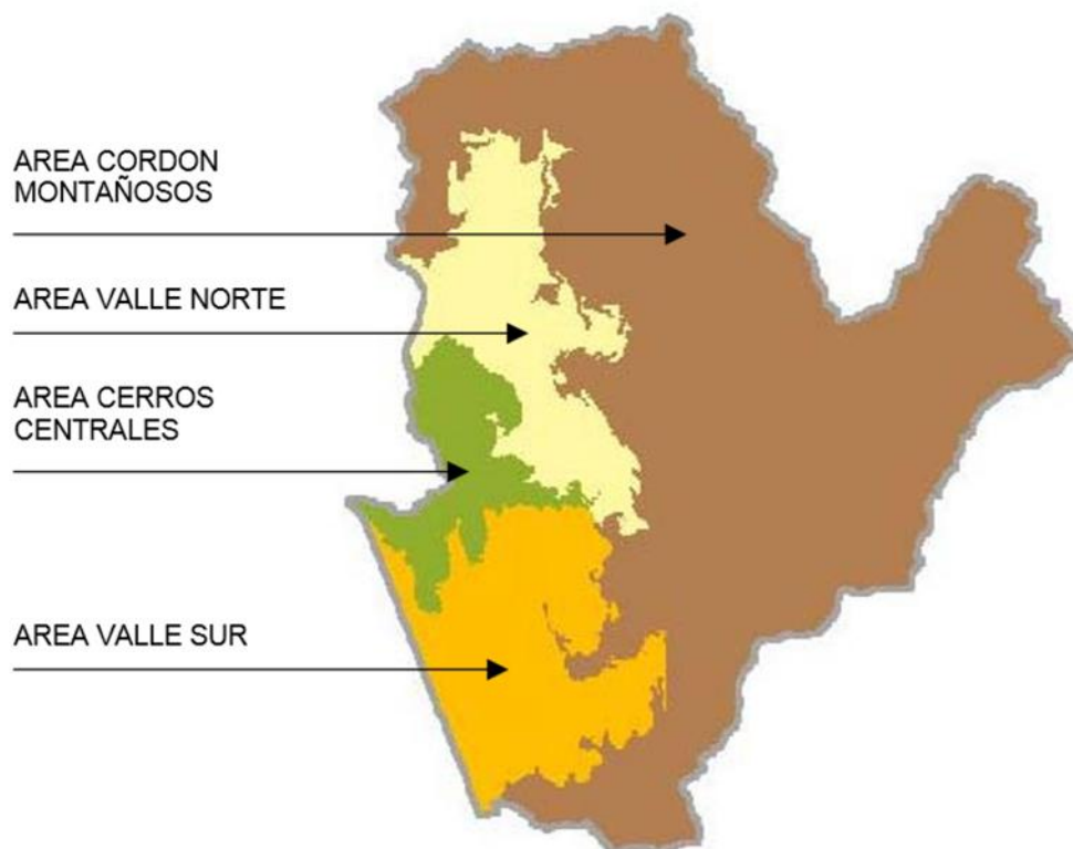
Imagen N°7: Esquema áreas geomorfológicas homogéneas Colina
