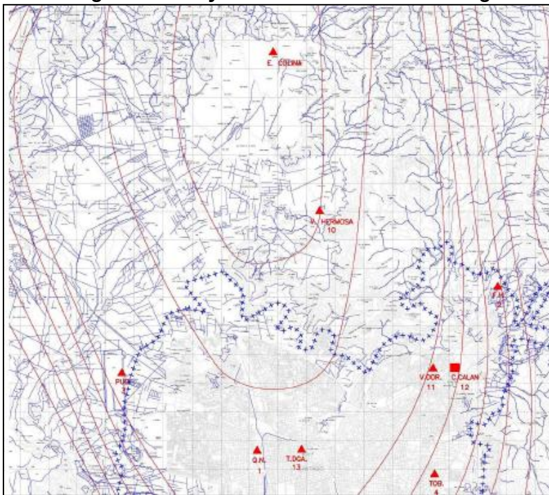
Imagen N°5: Isoyetas sector norte de Santiago
