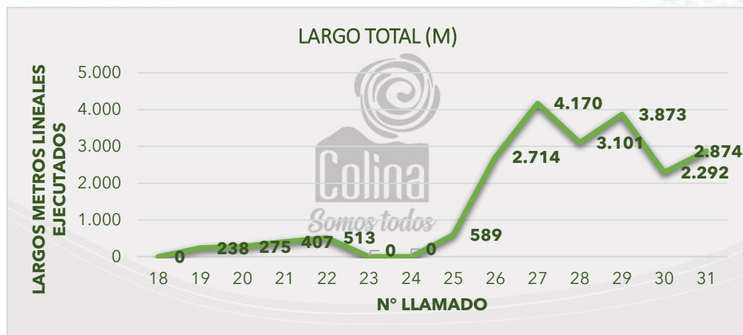
Proyección en Metros Lineales de pavimentación (2008 – 2021)
