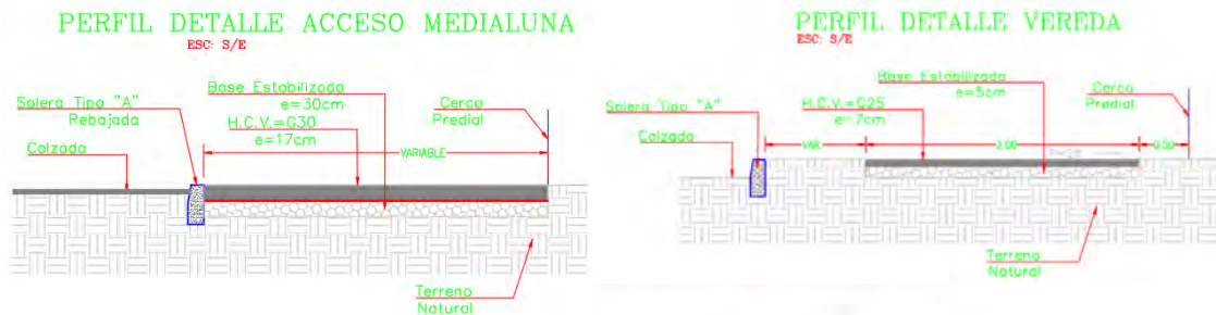
Perfil acceso vehicular, perfil veredas
