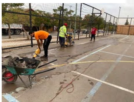
Trabajo de demarcación de carpeta asfáltica Los trabajos comienzan por retirar pavimento en mal estado y su reemplazo
